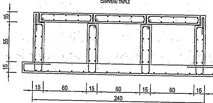
CANIVEAU TRIPLE
