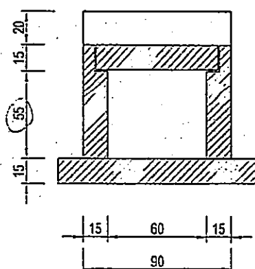
COUPE TRANSVERSALE
