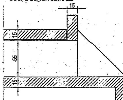
COUPE LONGITUDINALE
